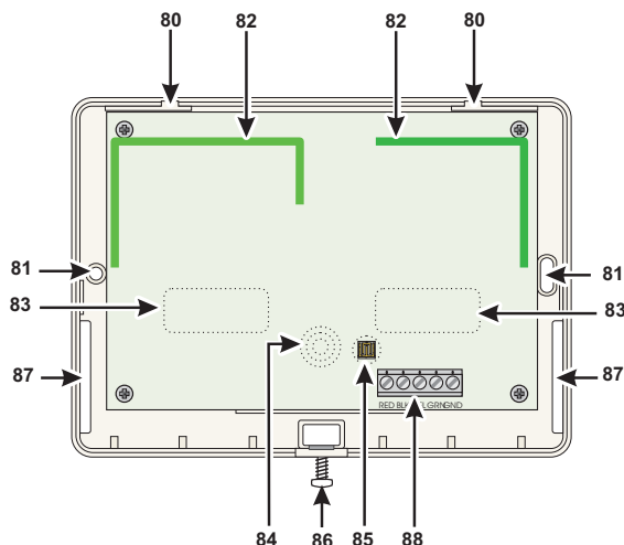
Figura 27 Parti del ricevitore.
