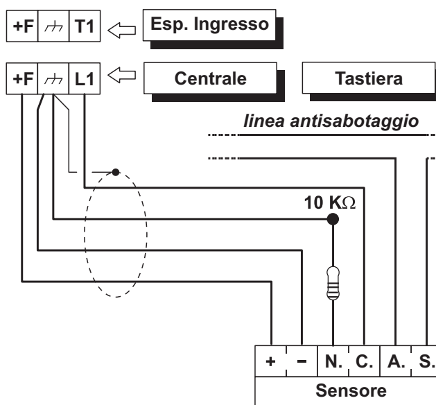
Figura 11 Collegamento di un sensore ad una Zona con Bilanciamento 10K o 10K solo allarme SEOL supervisione.
