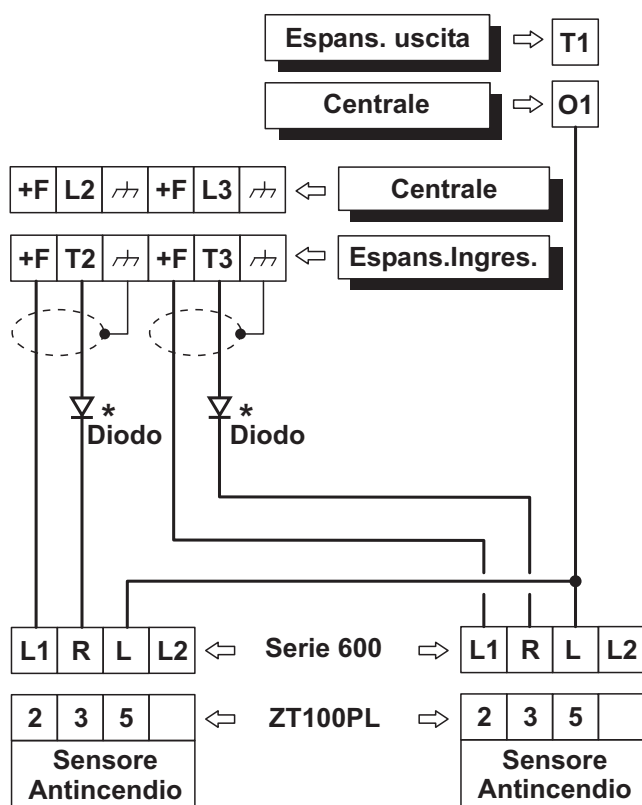
Figura 14 Collegamento di 2 sensori antincendio a Zone con Bilanciamento Normalmente Aperto (* Solo con la serie 600).
