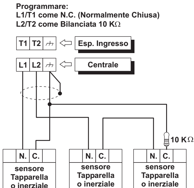
Figura 13 Collegamento di Sensori Inerziali (solo per le zone della Centrale) e Contatti per Tapparella: collegamento di un sensore ad una zona N.C. e di due sensori ad una zona Bilanciata 10K.
